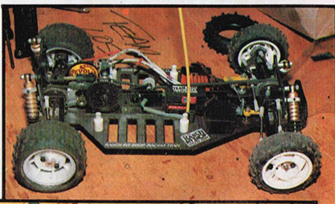
The unnamed new Yokomo.
